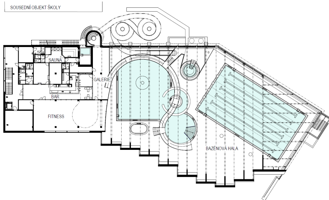
AQUAPARK KOHOUTOVICE PŮDORYS 2.NP
