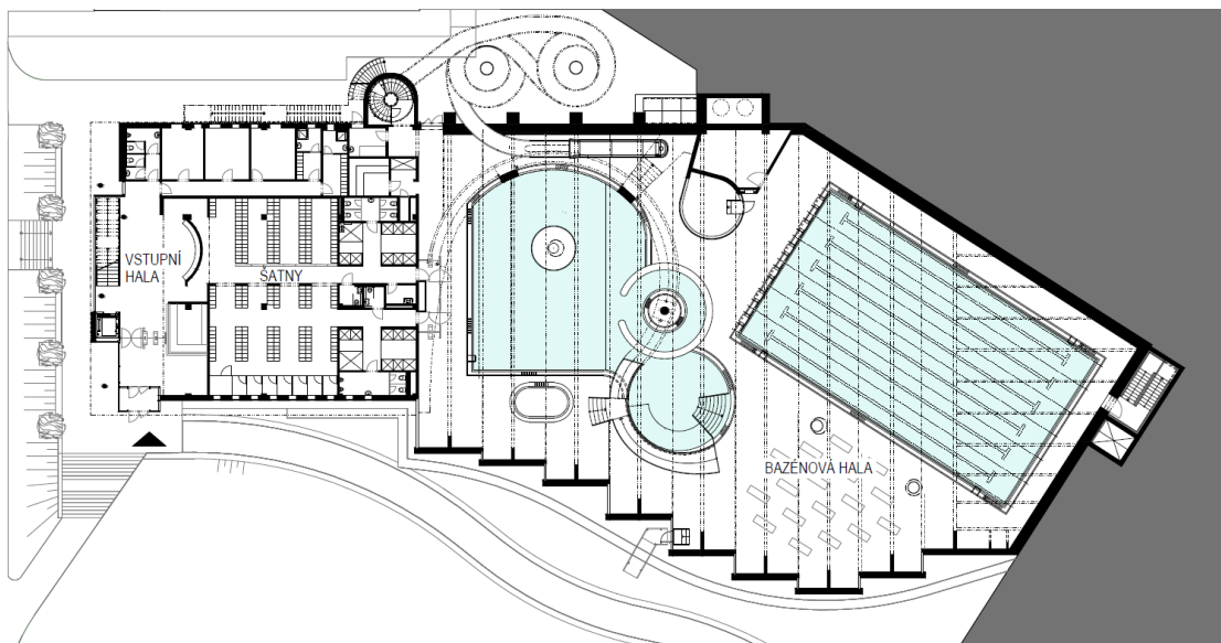
AQUAPARK KOHOUTOVICE PŮDORYS 2.NP
