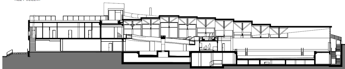
ŘEZ PODÉLNÝ
