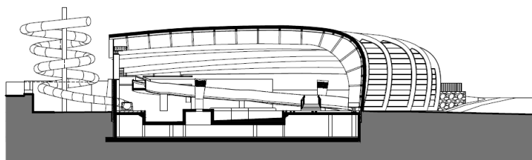
ŘEZ PRÍČNÝ
